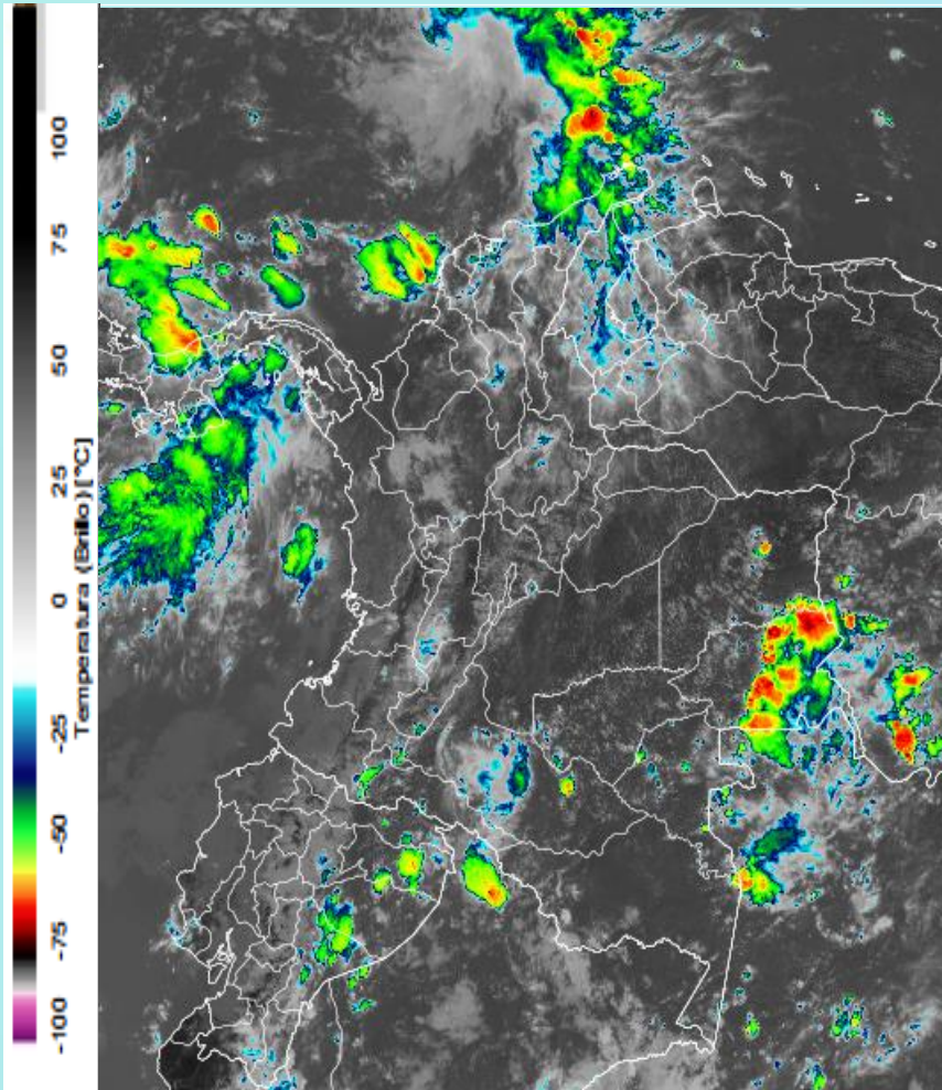
Imagen GOES East Canal Infrarrojo, 27 de noviembre de 2024 - Hora 12:00 HLC. Fuente: GOES 16
