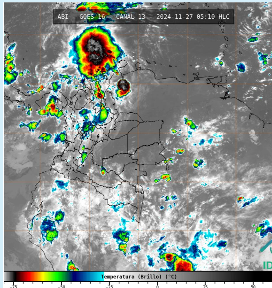
Imagen GOES 16 (East) Canal Infrarrojo | Fuente: GOES 16 - IDEAM 27 de noviembre de 2024 - Hora 05:10 HLC
