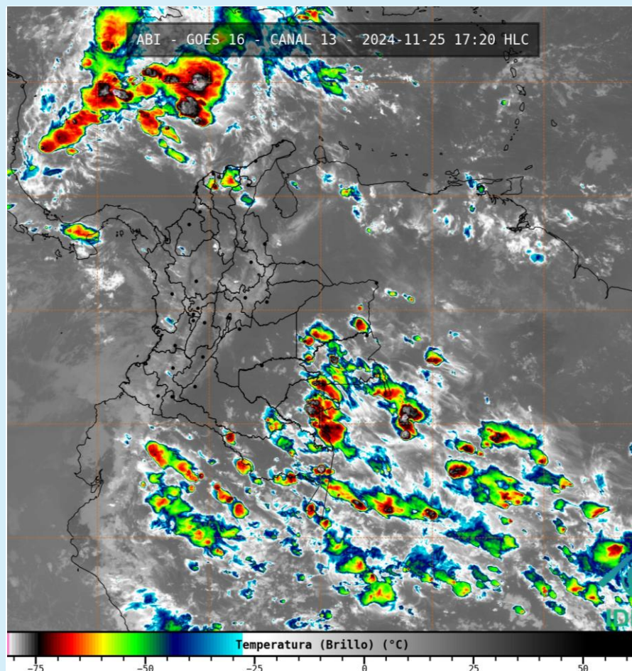
Imagen GOES 16 (East) Canal Infrarrojo | Fuente: GOES 16 - IDEAM 25 de noviembre de 2024 - Hora 17:20 HLC
