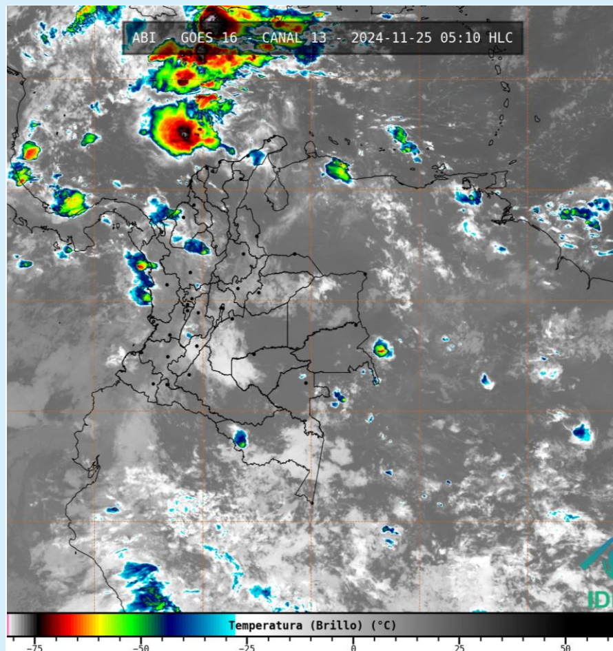
Imagen GOES 16 (East) Canal Infrarrojo | Fuente: GOES 16 - IDEAM 25 de noviembre de 2024 - Hora 05:10 HLC
