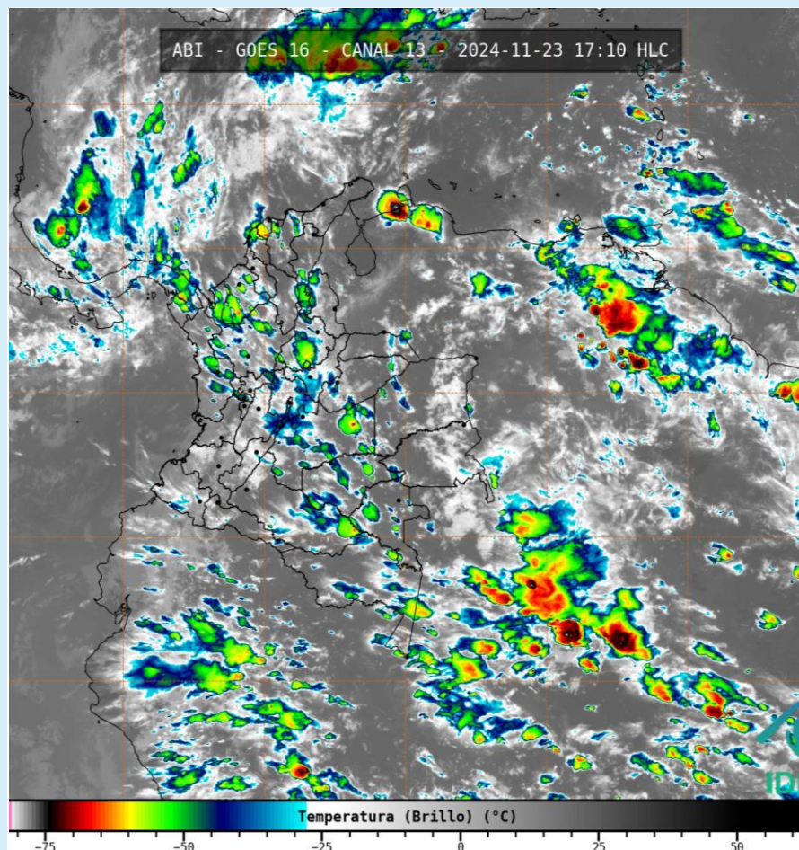
Imagen GOES 16 (East) Canal Infrarrojo | Fuente: GOES 16 - IDEAM 23 de noviembre de 2024 - Hora 17:10 HLC
