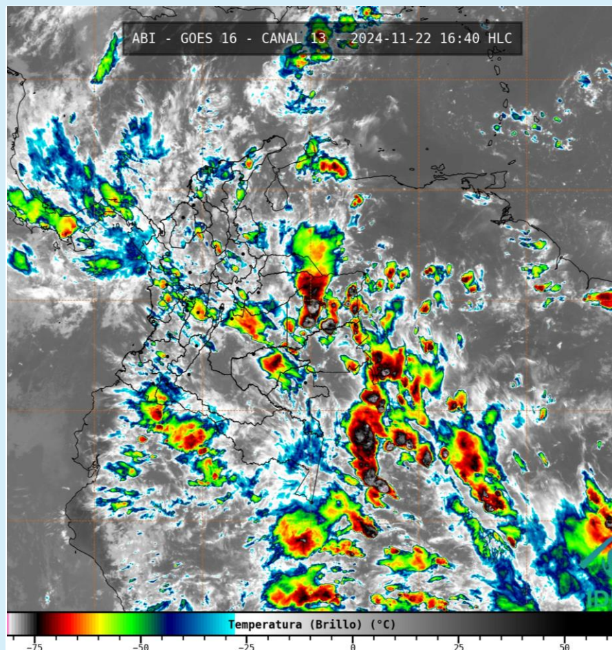
Imagen GOES 16 (East) Canal Infrarrojo | Fuente: GOES 16 - IDEAM 22 de noviembre de 2024 - Hora 16:40 HLC
