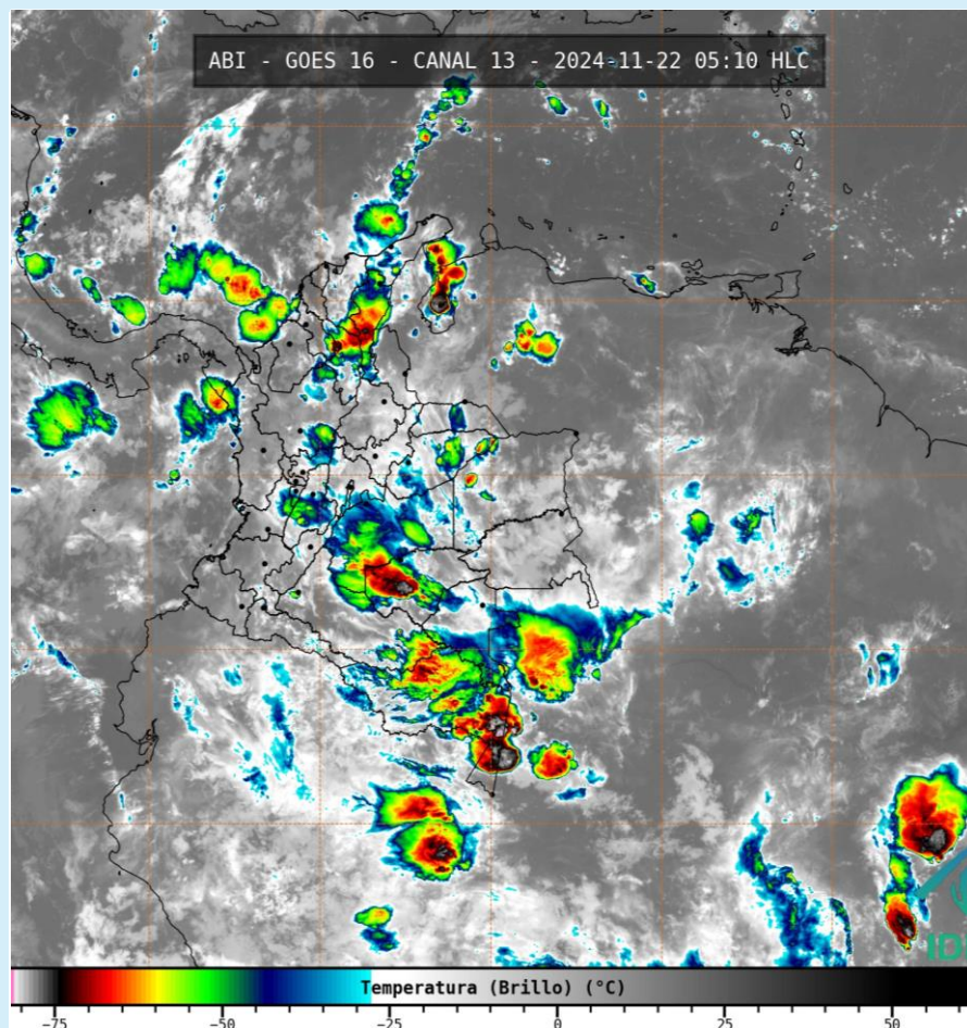
Imagen GOES 16 (East) Canal Infrarrojo | Fuente: GOES 16 - IDEAM 22 de noviembre de 2024 - Hora 05:10 HLC
