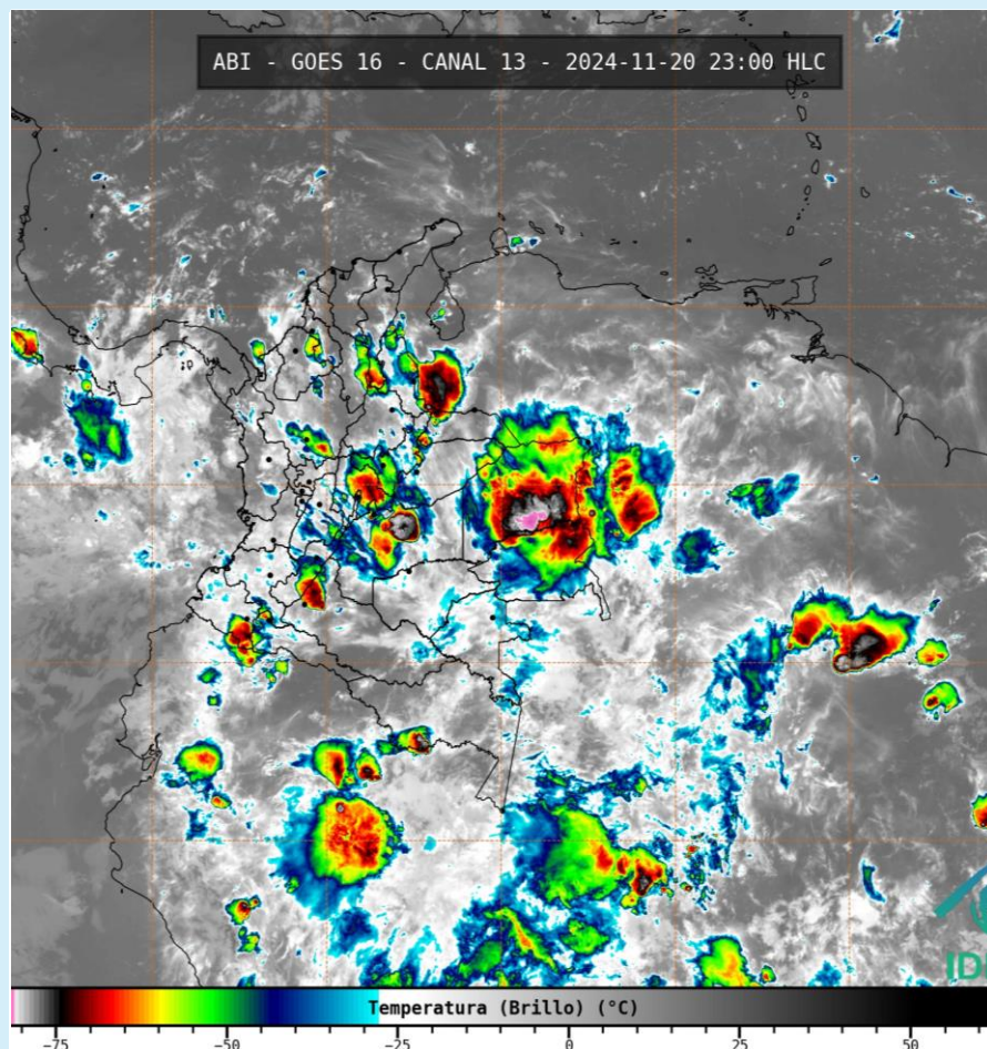
Imagen GOES 16 (East) Canal Infrarrojo | Fuente: GOES 16 - IDEAM 20 de noviembre de 2024 - Hora 23:00 HLC
