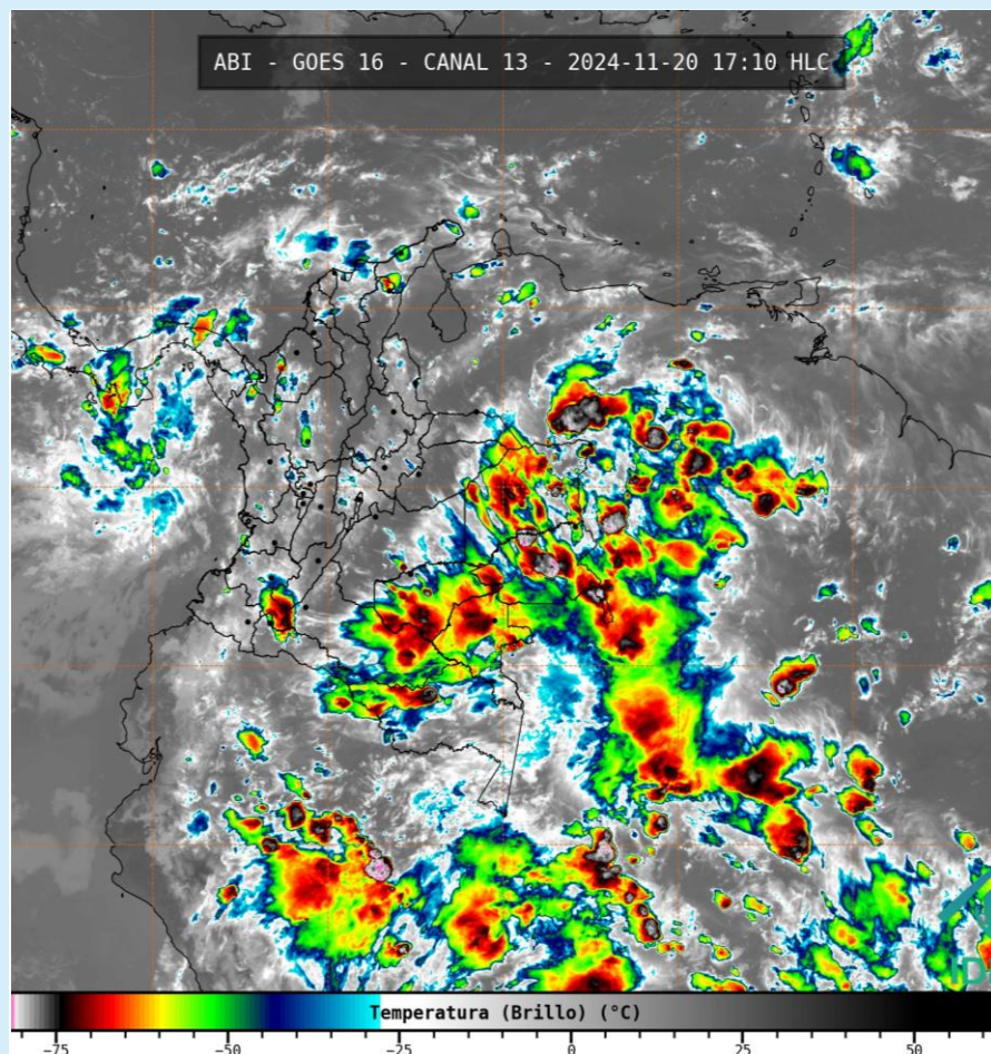
Imagen GOES 16 (East) Canal Infrarrojo | Fuente: GOES 16 - IDEAM 20 de noviembre de 2024 - Hora 17:10 HLC
