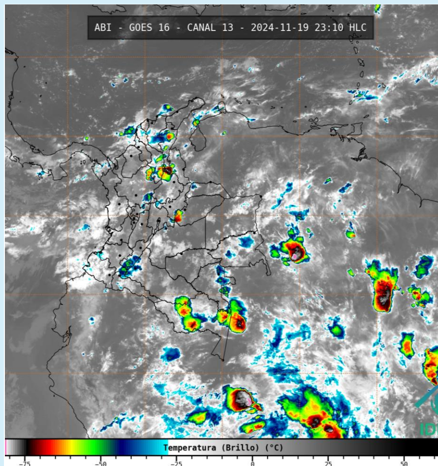
Imagen GOES 16 (East) Canal Infrarrojo | Fuente: GOES 16 - IDEAM 19 de noviembre de 2024 - Hora 23:10 HLC
