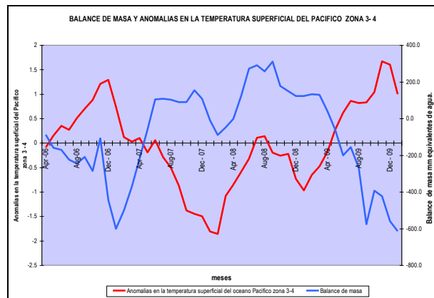
Gráfica 21. Balance de masa y anomalías en la temperatura superficial del océano Pacífico región 3 - 4.
