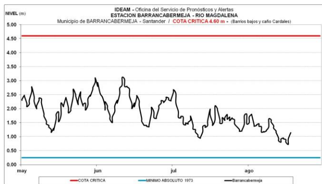
Gráfica No 11. Niveles del río Magdalena en Barrancabermeja (Santander)
