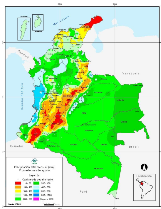
Mapa N° 1. Promedio histórico de la precipitación para el mes de agosto.
