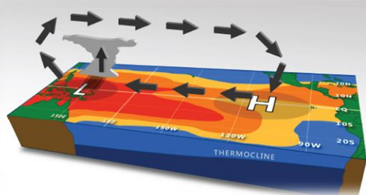
Gráfica N° 1. Condiciones NEUTRALES sobre la cuenca del Océano Pacífico tropical. Temperaturas bajas en tonos azules; temperaturas altas en colores entre naranjas a rojos. Tomado de:
