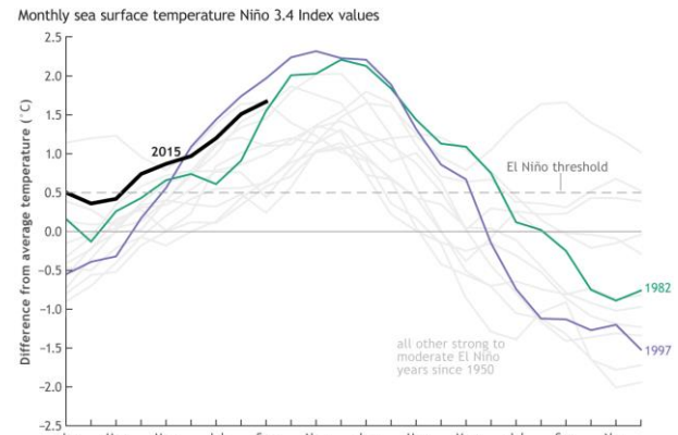
Gráfica N° 3a. Comparación de anomalías de la temperatura superficial del mar en la región Niño 3.4 del Pacífico tropical. Tomado de: http://www.cpc.ncep.noaa.gov/products/
