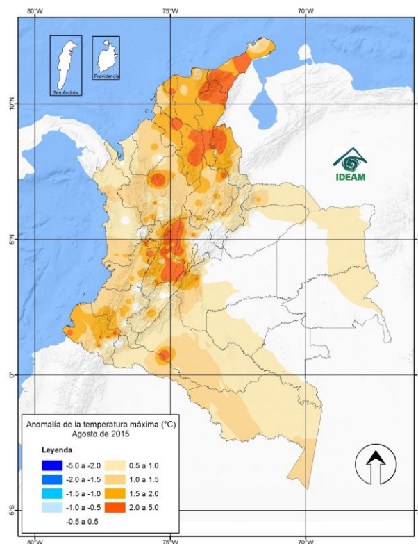
Mapa N° 3. Anomalías de la temperatura MÁXIMA en agosto de 2015.
