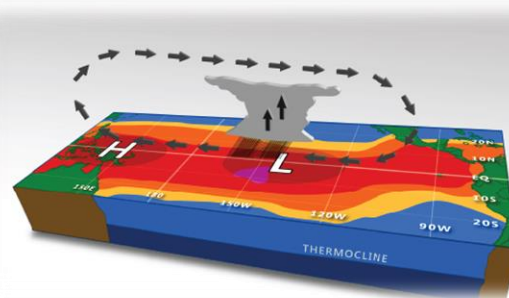
Gráfica N° 2. Condiciones oceano-atmosféricas bajo un evento EL NIÑO sobre la cuenca del Océano Pacífico tropical. Temperaturas bajas de en tonos azules; temperaturas altas en colores entre naranjas a rojos. Tomado de:
