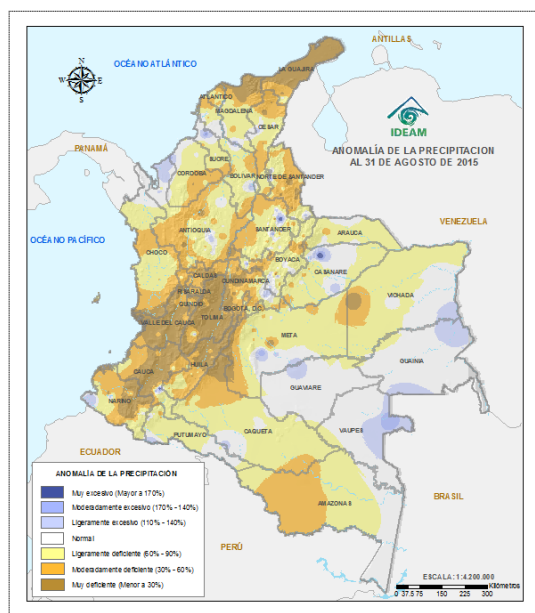
Mapa N° 2. Anomalías de la precipitación para el mes de agosto de 2015, con respecto al promedio histórico de agosto (serie 1981-2010).
