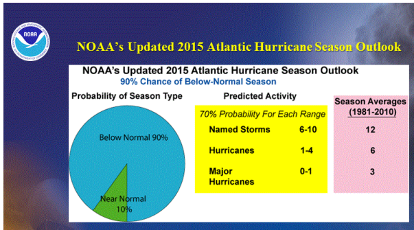
Grafica No 4. Predicciones de la NOAA para la temporada de huracanes en el Atlántico 2015. Fuente: http://www.nhc.noaa.gov/climo/
