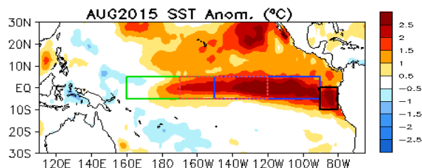
Gráfica N° 3. Mapa de anomalías de temperatura superficial del mar en el Océano Pacífico Tropical para el mes de agosto de 2015. Los valores de las anomalías por debajo de los promedios para la época se presentan en tonos azules; por encima de la media para la época en colores amarillos a rojos. Tomado de: http://www.cpc.ncep.noaa.gov/products/
