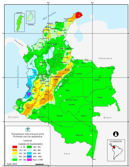
Mapa No 4. Precipitación total mensual promedio para el mes de septiembre.
