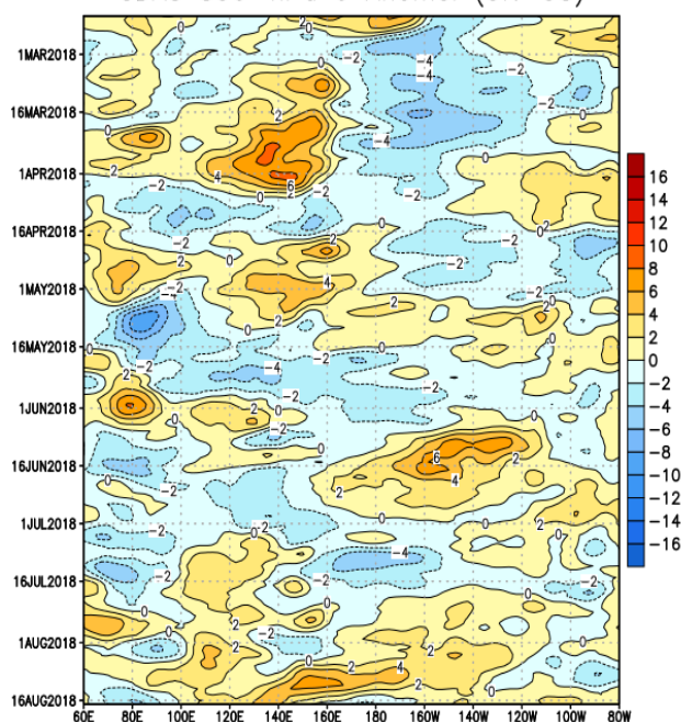
Figura 3. Evolución en el tiempo de las anomalías del viento en niveles bajos de la atmósfera (850 mb, aprox 1500 snm) entre 5°N y 5°S, para los meses de marzo a agosto de 2018. Las áreas sombreadas muestran las evoluciones en el tiempo de anomalías de viento del Este (colores azules) y del Oeste (vientos del oeste).
