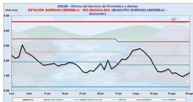
Figura 13. Niveles del río Magdalena en Barrancabermeja (Santander)
