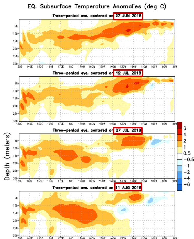
Figura 2. Evolución de las anomalías de la Temperatura Subsuperficial del Mar – TSSM en el océano Pacífico tropical, entre el 27 de junio y el 11 de agosto de 2018.
