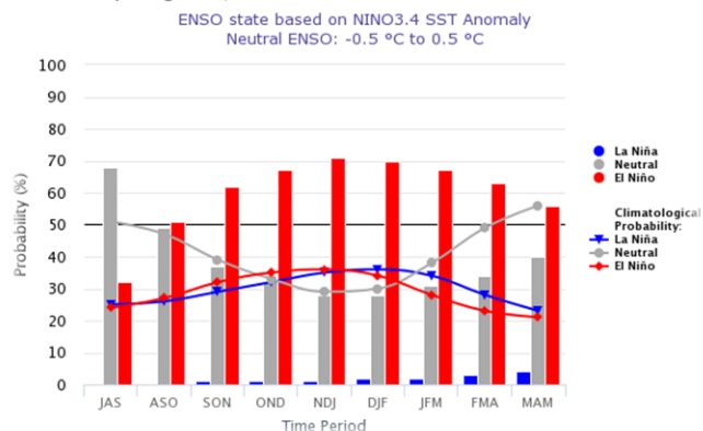
Figura 5. Probabilidad de desarrollo de fenómenos Niño/Niña, basados en la proyección de anomalías de la temperatura superficial del mar para la Región Niño 3.4 en el océano Pacífico tropical, entre los meses de agosto de 2018 y abril de 2019. Las barras azules indican probabilidad en condiciones frías (asociadas con un fenómeno La Niña), las barras grises indican probabilidad de prevalencia de condiciones neutrales y las barras rojas indican probabilidad de calentamiento (asociadas con un fenómeno El Niño). Fuente: International Research Institute for Climate and Society. goq.gl/KoRqmE
