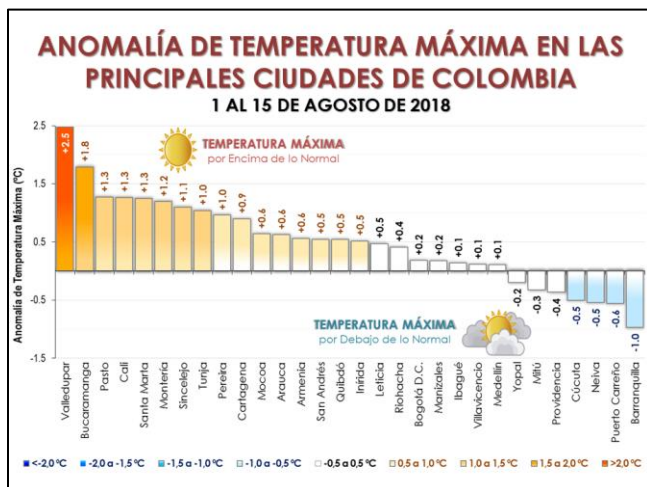
Figura 9. Anomalía de temperatura máxima para las principales ciudades del país durante los primeros 15 días del mes de agosto de 2018. Fuente: IDEAM
