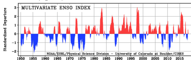
Figura 4. Comportamiento del índice MEI entre 1950 y 2018. Una clara persistencia de colores rojos indica asociación con fenómenos El Niño históricos, mientras que los de color azul se asocian a fenómenos La Niña. Fuente: http://www.esrl.noaa.gov
