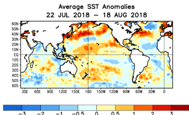
Figura 1. Mapa del promedio de las Anomalías semanales de la Temperatura Superficial del Mar – ATSM, en el Océano Pacífico Tropical durante el último mes (entre el 22 de julio y el 18 de agosto de 2018). Los valores de las anomalías por debajo de los promedios para la época se presentan en tonos azules, mientras que aquellos que se muestran en colores amarillos a rojos, representan valores por encima de la media para la época. Tomado de:
