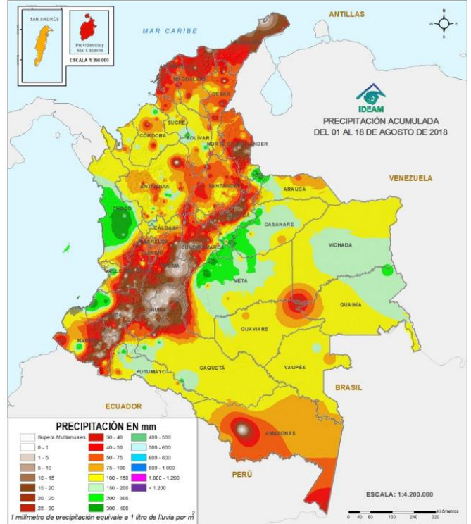
Figura 8. Precipitación total acumulada entre el 1 y el 18 de agosto de 2018. Fuente: IDEAM
