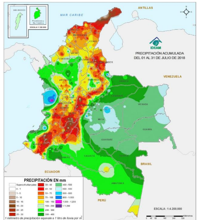
Figura 7. Precipitación total acumulada para el mes de julio de 2018. Fuente: IDEAM.
