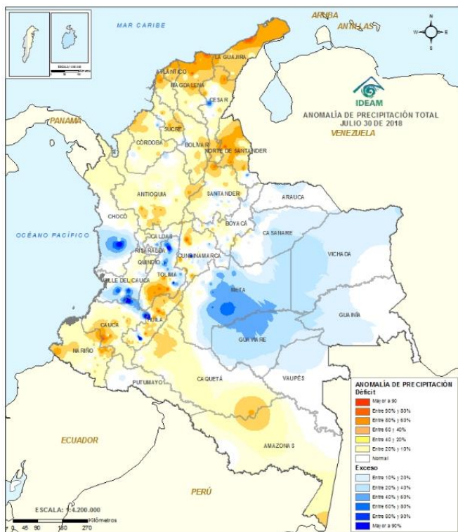
Figura 6. Anomalías de la precipitación para el mes de julio de 2018, con respecto a su promedio histórico (serie 1981-2010). Fuente: IDEAM.
