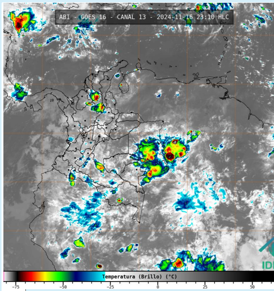
Imagen GOES 16 (East) Canal Infrarrojo | Fuente: GOES 16 - IDEAM 16 de noviembre de 2024 - Hora 23:10 HLC
