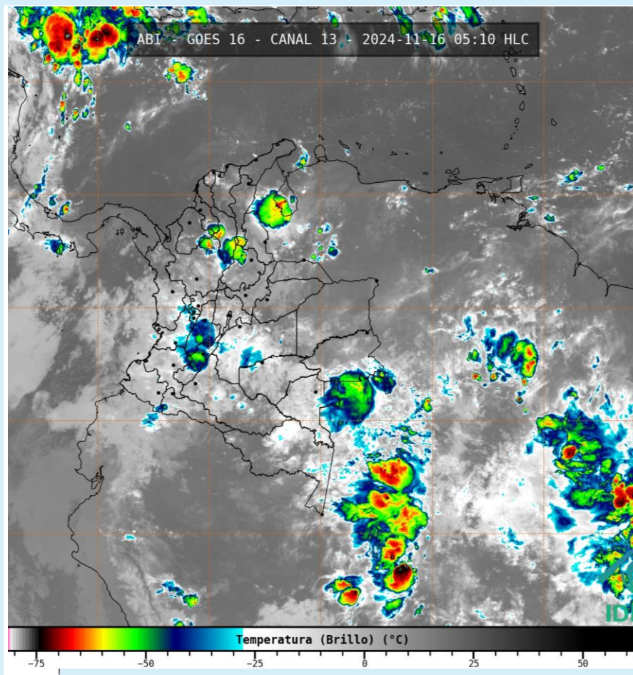
Imagen GOES 16 (East) Canal Infrarrojo | Fuente: GOES 16 - IDEAM 16 de noviembre de 2024 - Hora 05:10 HLC
