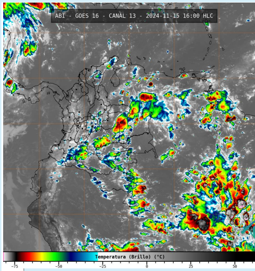
Imagen GOES 16 (East) Canal Infrarrojo | Fuente: GOES 16 - IDEAM 15 de noviembre de 2024 - Hora 16:00 HLC
