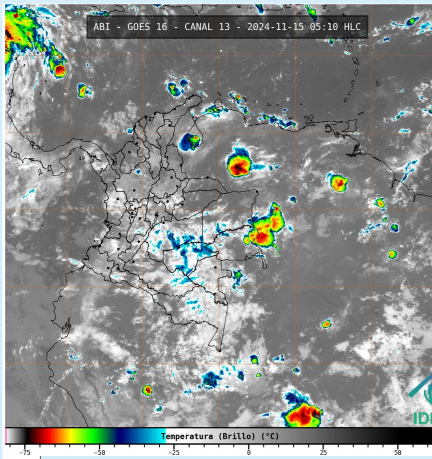
Imagen GOES 16 (East) Canal Infrarrojo | Fuente: GOES 16 - IDEAM 15 de noviembre de 2024 - Hora 05:10 HLC
