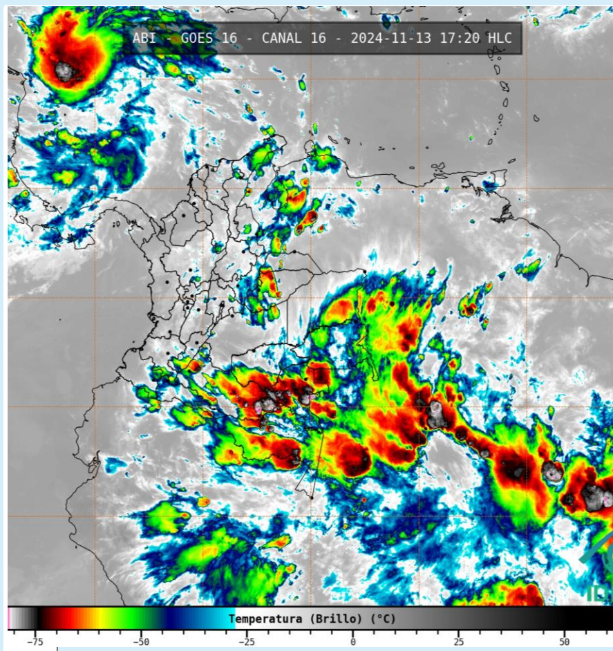
Imagen GOES 16 (East) Canal Infrarrojo | Fuente: GOES 16 - IDEAM 13 de noviembre de 2024 - Hora 17:20 HLC
