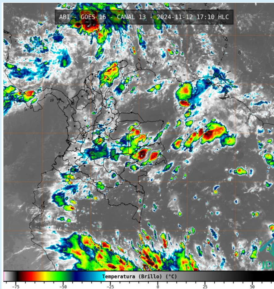
Imagen GOES 16 (East) Canal Infrarrojo | Fuente: GOES 16 - IDEAM 12 de noviembre de 2024 - Hora 17:10 HLC
