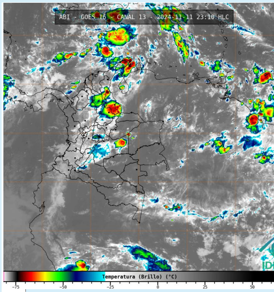
Imagen GOES 16 (East) Canal Infrarrojo | Fuente: GOES 16 - IDEAM 11 de noviembre de 2024 - Hora 23:00 HLC
