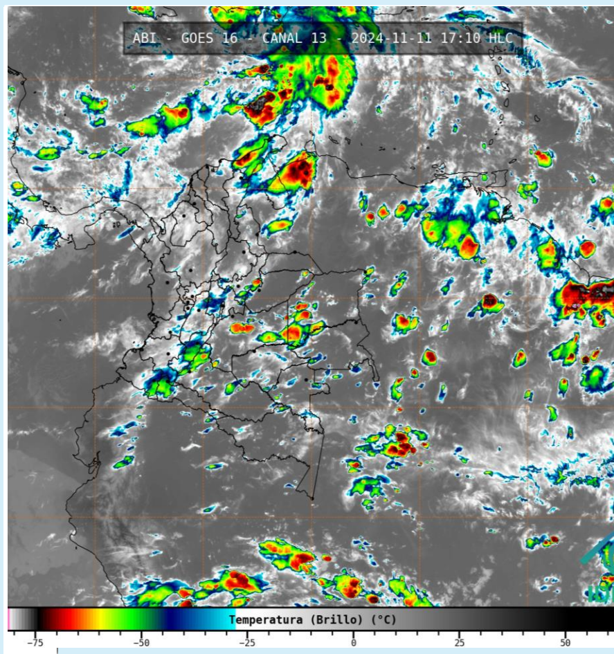
Imagen GOES 16 (East) Canal Infrarrojo | Fuente: GOES 16 - IDEAM 11 de noviembre de 2024 - Hora 17:10 HLC
