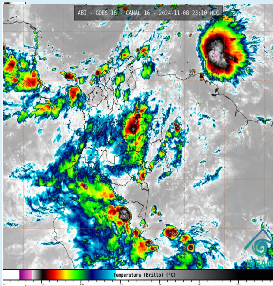
Imagen GOES 16 (East) Canal Infrarrojo | Fuente: GOES 16 - IDEAM 8 de noviembre de 2024 - Hora 23:10 HLC
