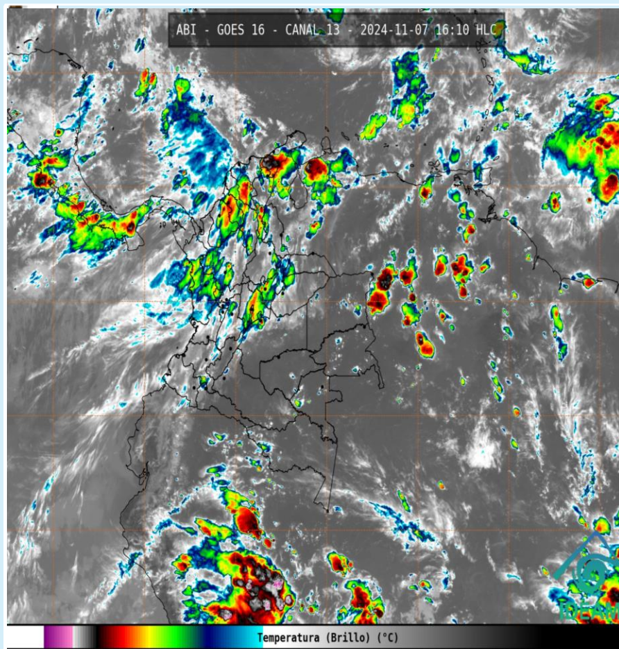
Imagen GOES 16 (East) Canal Infrarrojo | Fuente: GOES 16 - IDEAM 7 de noviembre de 2024 - Hora 16:10 HLC
