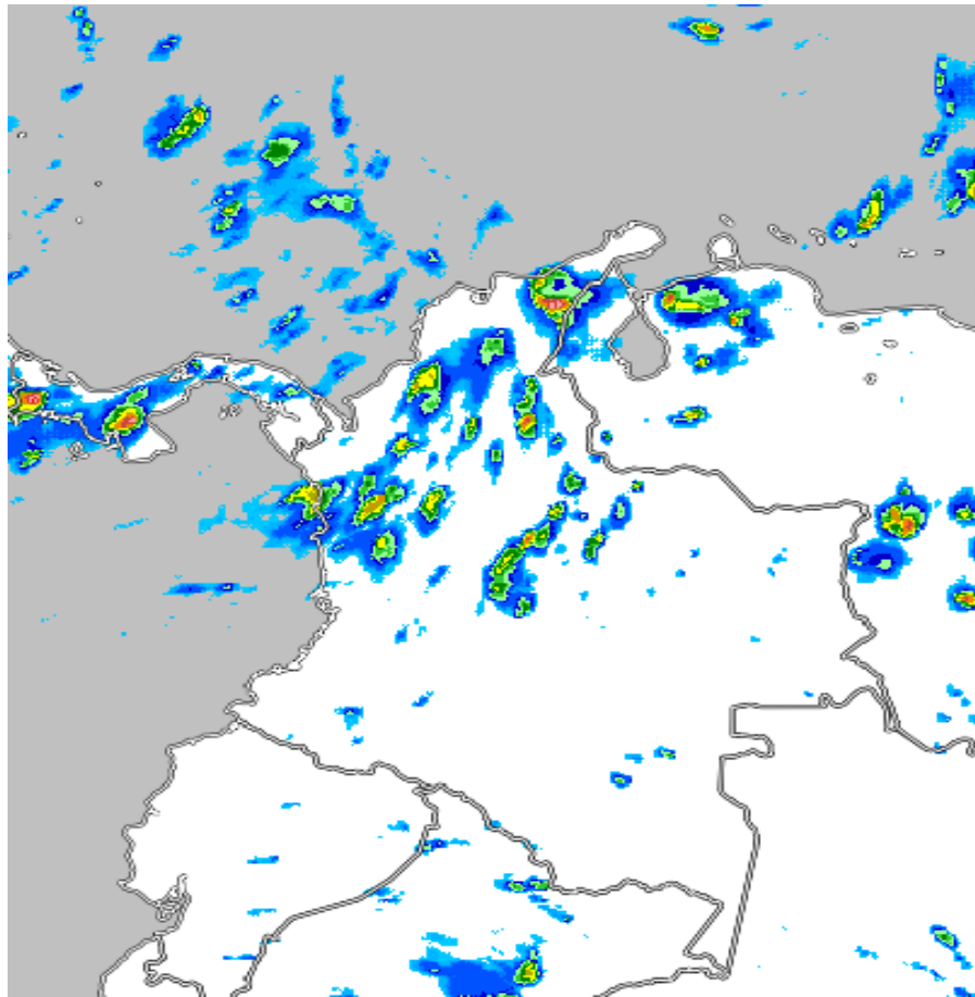
Hidroestimador últimas 06 horas Fuente: NESDIS-NOAA
