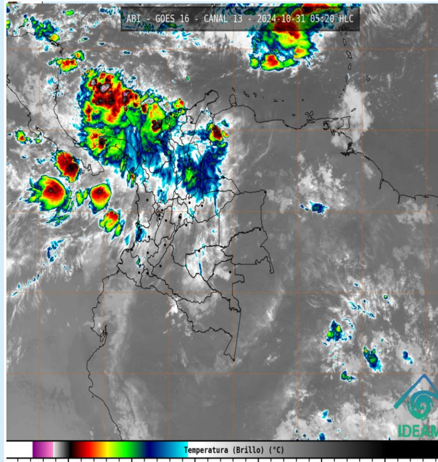
Imagen GOES 16 (East) Canal Infrarrojo | Fuente: GOES 16 - IDEAM 31 de octubre de 2024 - Hora 05:20 HLC
