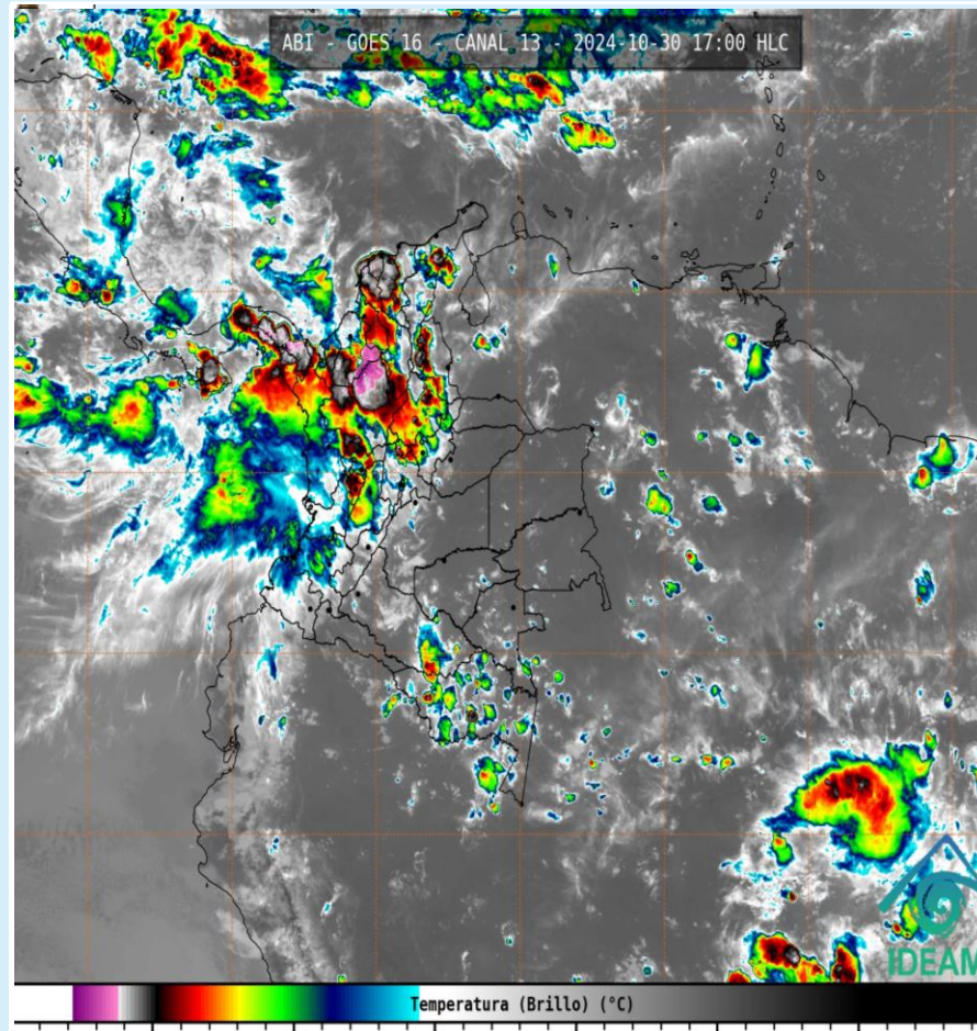
Imagen GOES 16 (East) Canal Infrarrojo | Fuente: GOES 16 - IDEAM 30 de octubre de 2024 - Hora 17:00 HLC
