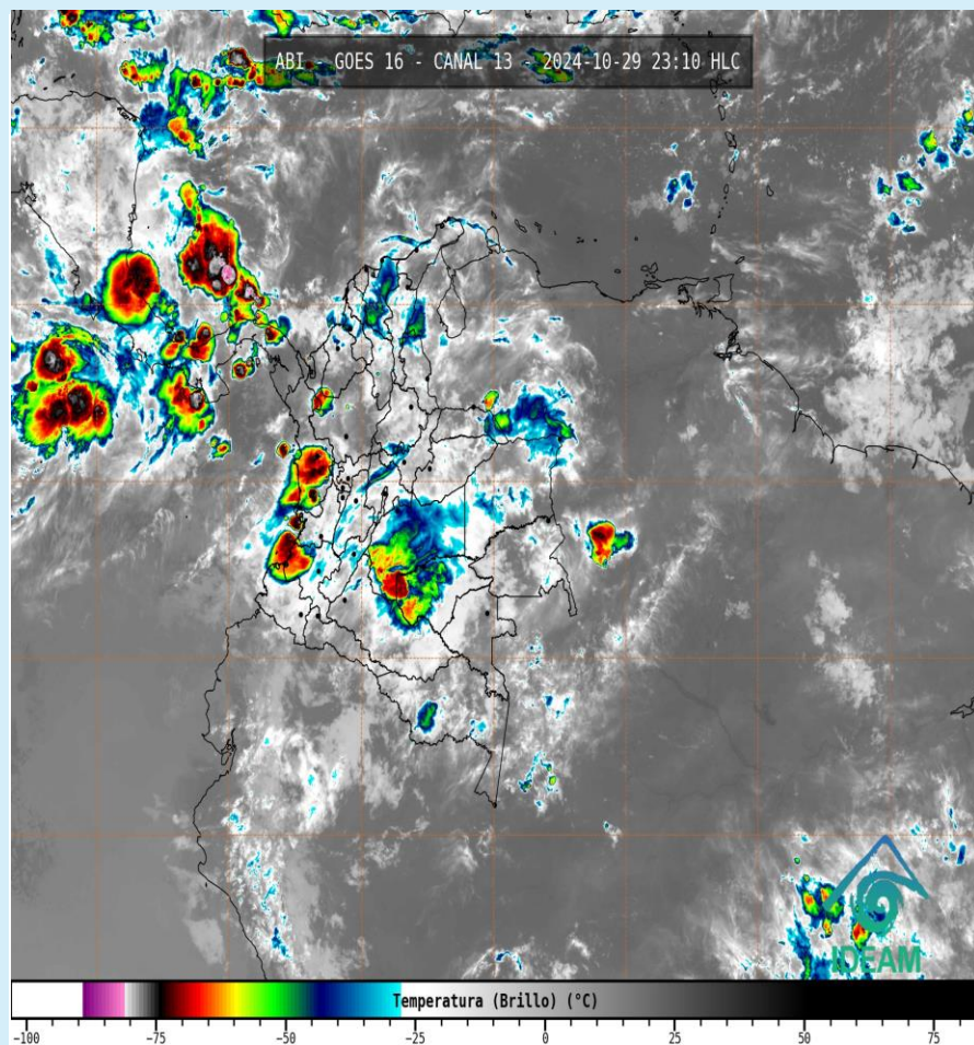
Imagen GOES 16 (East) Canal Infrarrojo | Fuente: RAMMB 29 de octubre de 2024 - Hora 23:10 HLC
