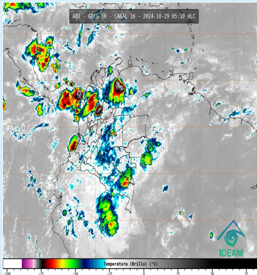
Imagen GOES 16 (East) Canal Infrarrojo | Fuente: IDEAM – GOES16 29 de octubre de 2024 - Hora 05:10 HLC
