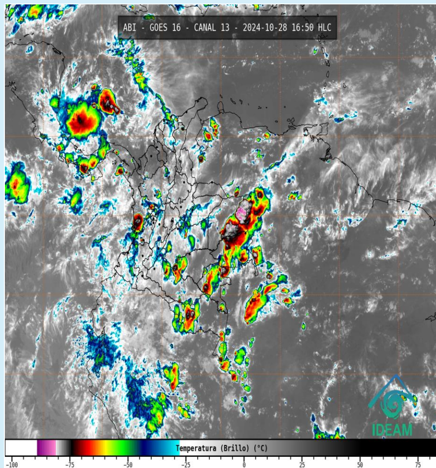
Imagen GOES 16 (East) Canal Infrarrojo | Fuente: IDEAM – GOES16 28 de octubre de 2024 - Hora 16:50 HLC
