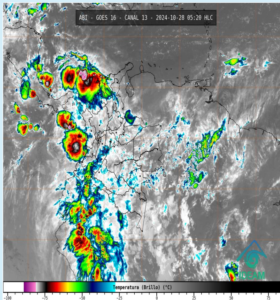
Imagen GOES 16 (East) Canal Infrarrojo | Fuente: IDEAM – GOES16 28 de octubre de 2024 - Hora 05:20 HLC
