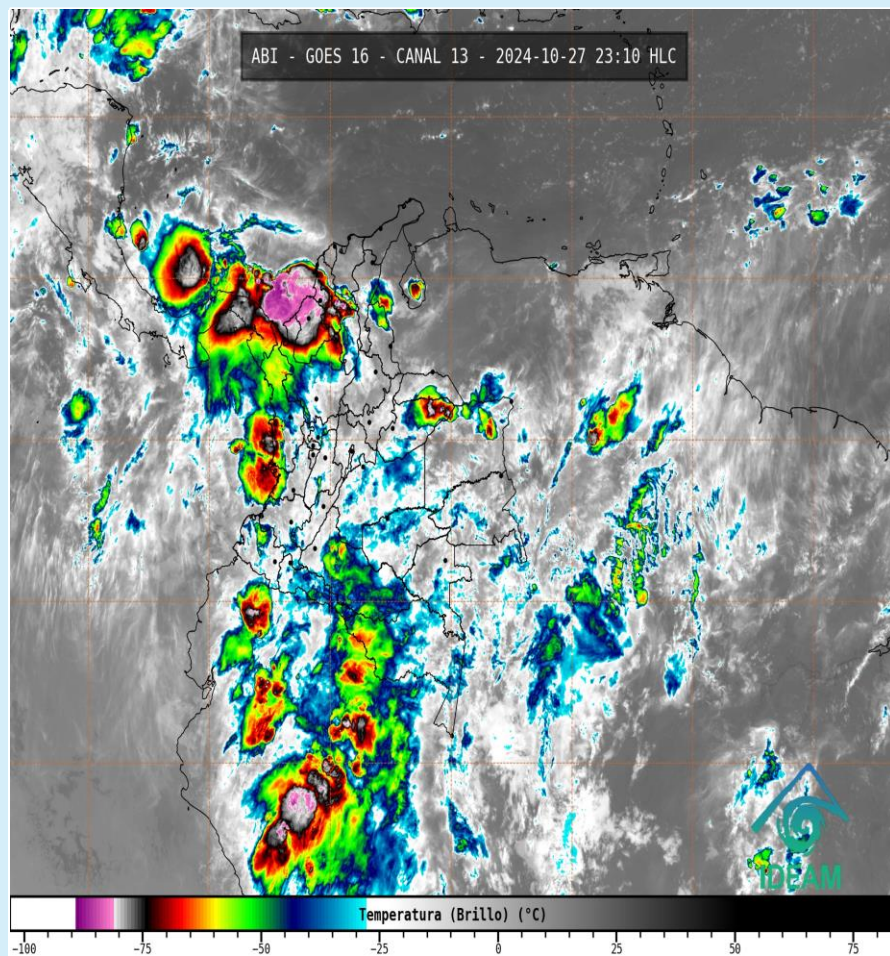
Imagen GOES 16 (East) Canal Infrarrojo | Fuente: IDEAM – GOES16 27 de octubre de 2024 - Hora 23:10 HLC
