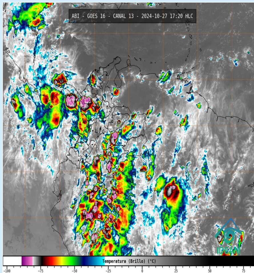
Imagen GOES 16 (East) Canal Infrarrojo | Fuente: IDEAM – GOES16 27 de octubre de 2024 - Hora 17:20 HLC
