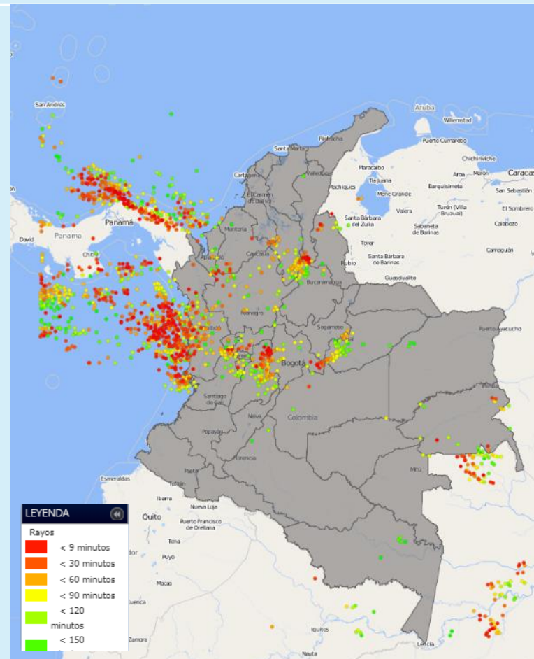
Descargas eléctricas en las últimas 3 horas Fuente: Keraunos
