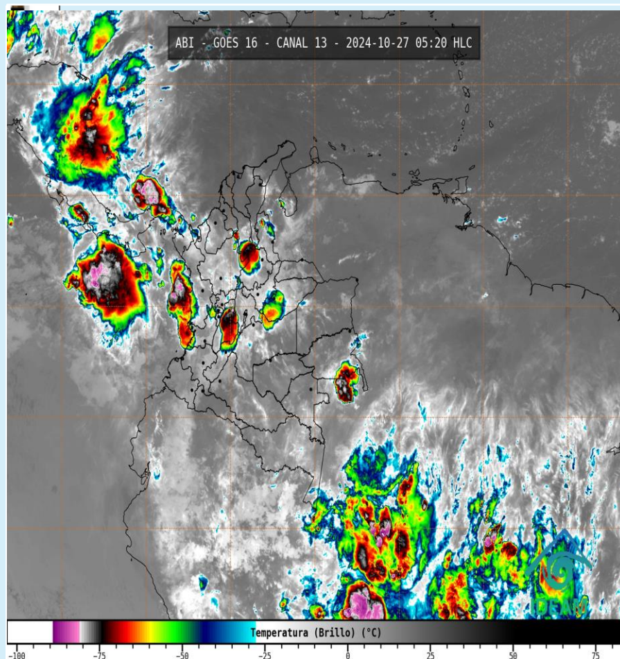
Imagen GOES 16 (East) Canal Infrarrojo | Fuente: IDEAM – GOES16 27 de octubre de 2024 - Hora 05:20 HLC
