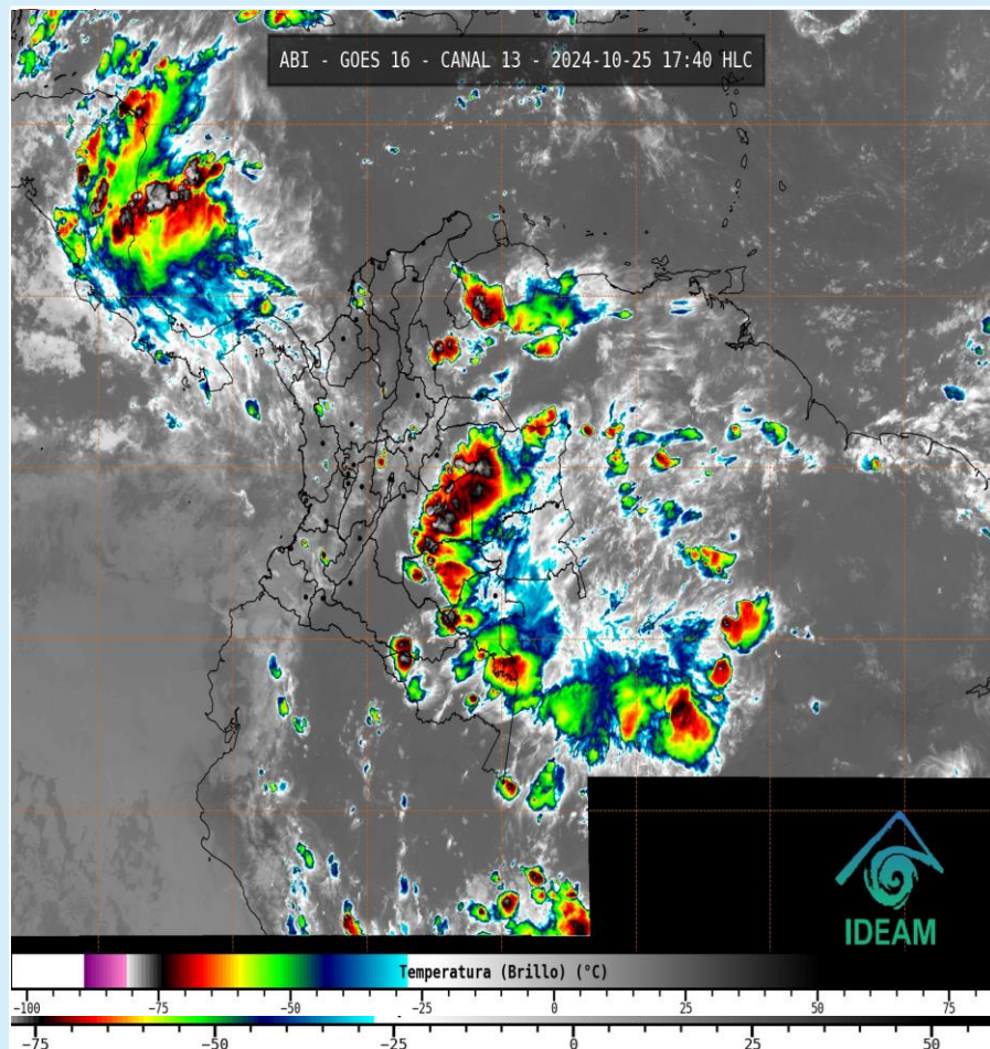
Imagen GOES 16 (East) Canal Infrarrojo | 25 de octubre de 2024 – Hora 17:40 HLC Fuente: GOES 16 - IDEAM
