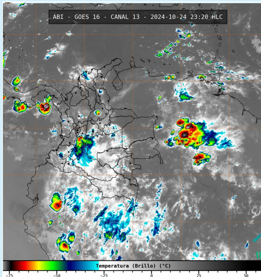
Imagen GOES 16 (East) Canal Infrarrojo | 25 de octubre de 2024 – Hora 23:20 HLC Fuente: GOES 16 - IDEAM
