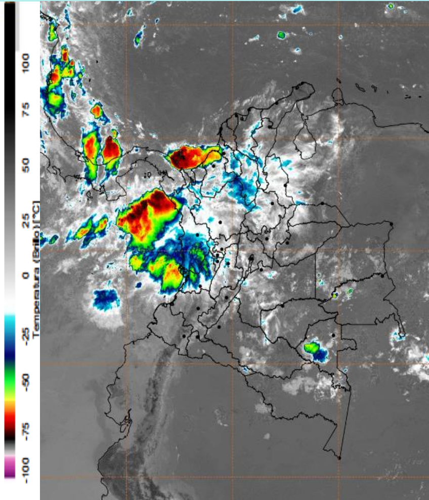
Imagen GOES East Canal Infrarrojo, 19 de octubre de 2024 - Hora 11:30 HLC. Fuente: GOES 16
