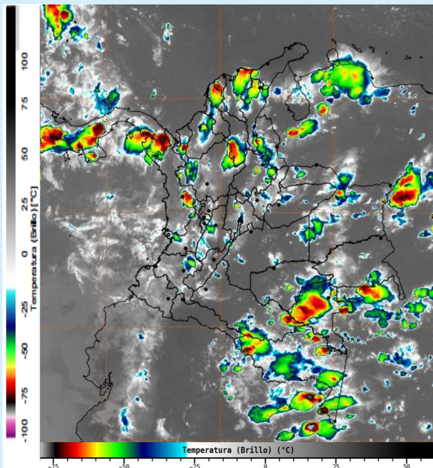
Imagen GOES 16 (East) Canal Infrarrojo | 18 de octubre de 2024 – Hora 17:10 HLC Fuente: GOES 16 - IDEAM
