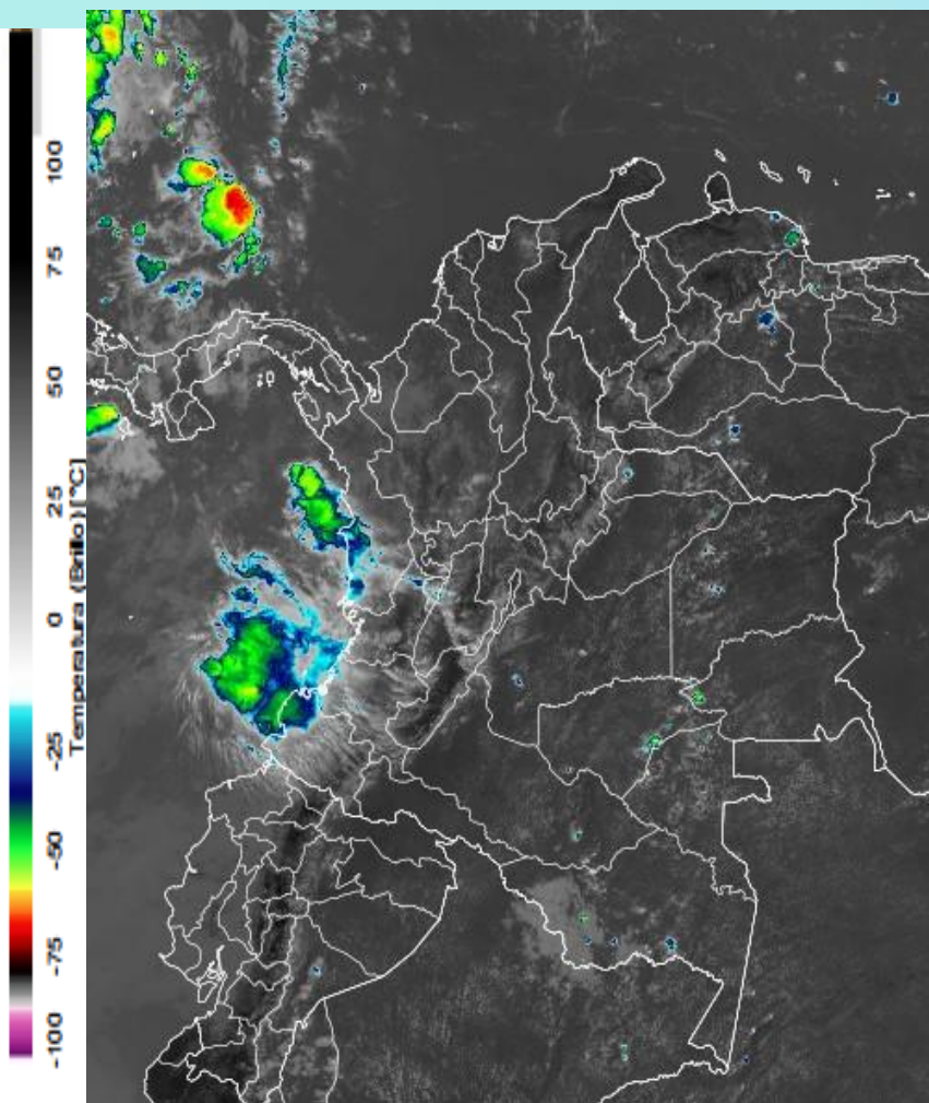
Imagen GOES East Canal Infrarrojo, 18 de octubre de 2024 - Hora 11:40 HLC. Fuente: GOES 16
