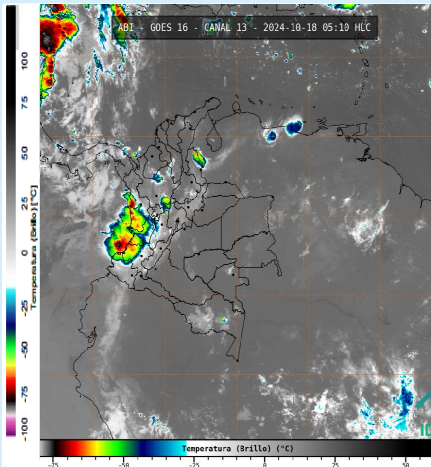
Imagen GOES 16 (East) Canal Infrarrojo | 18 de octubre de 2024 – Hora 05:10 HLC Fuente: GOES 16 - IDEAM
