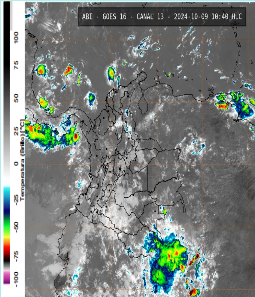
Imagen GOES East Canal Infrarrojo, 9 de octubre de 2024 - Hora 10:40 HLC. Fuente: GOES 16
