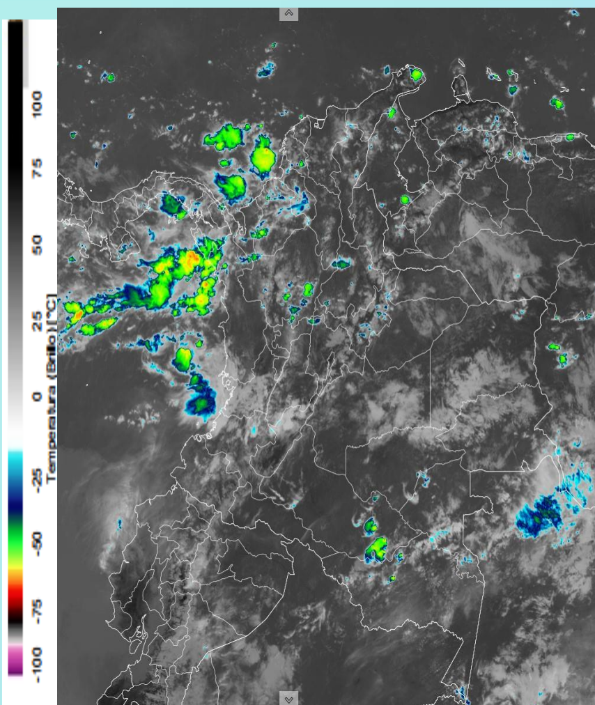
Imagen GOES East Canal Infrarrojo, 7 de octubre de 2024 - Hora 11:40 HLC. Fuente: GOES 16
