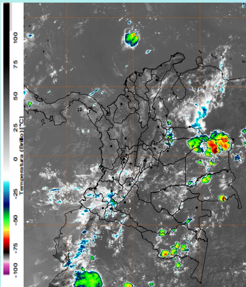
Imagen GOES East Canal Infrarrojo, 3 de octubre de 2024 - Hora 12:10 HLC. Fuente: GOES 16
