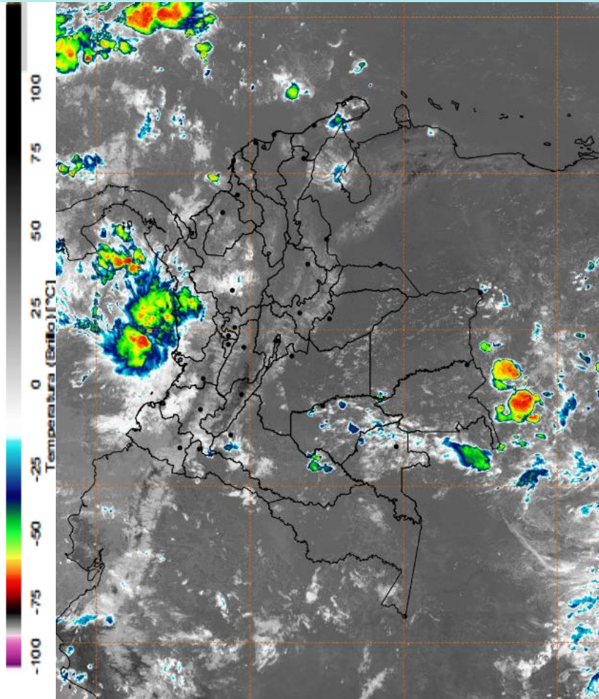
Imagen GOES East Canal Infrarrojo, 1 de octubre de 2024 - Hora 11:30 HLC. Fuente: GOES 16
