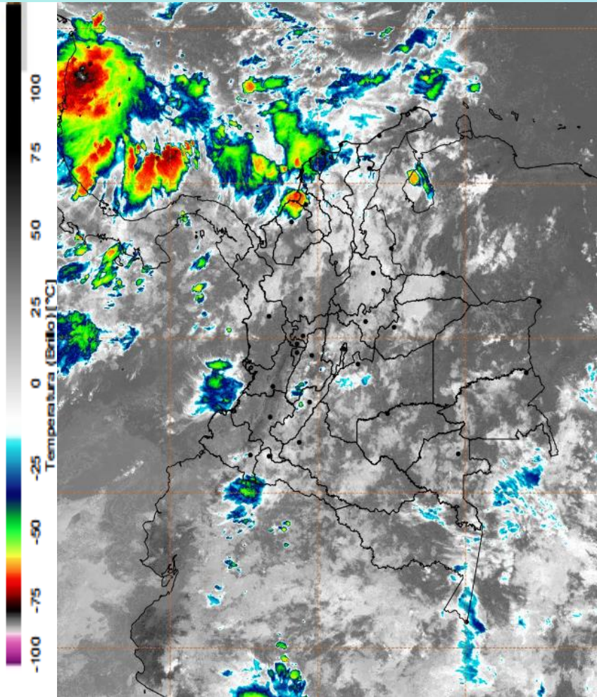
Imagen GOES East Canal Infrarrojo, 30 de septiembre de 2024 - Hora 11:30 HLC. Fuente: GOES 16
