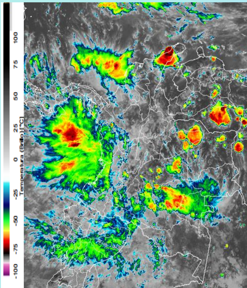
Imagen GOES East Canal Infrarrojo, 28 de septiembre de 2024 - Hora 12:00 HLC. Fuente: GOES 16
