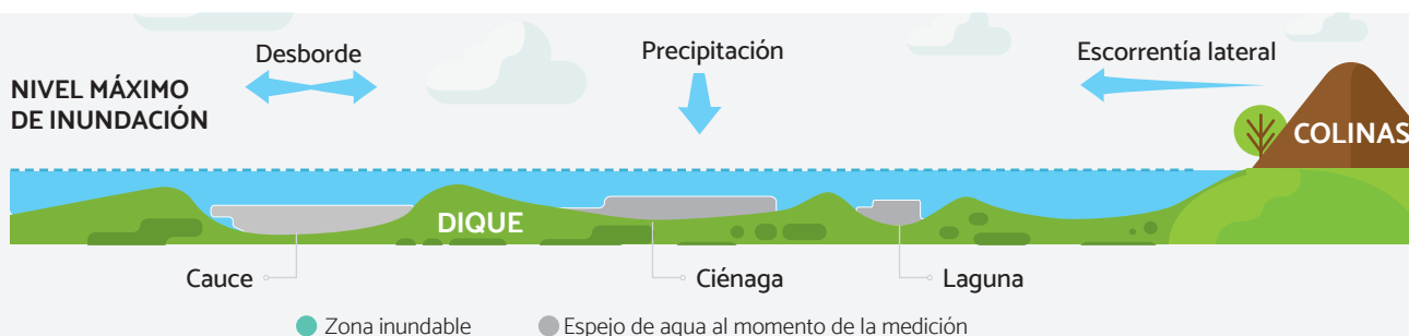
• Figura 31. Representación general de una zona inundable.
