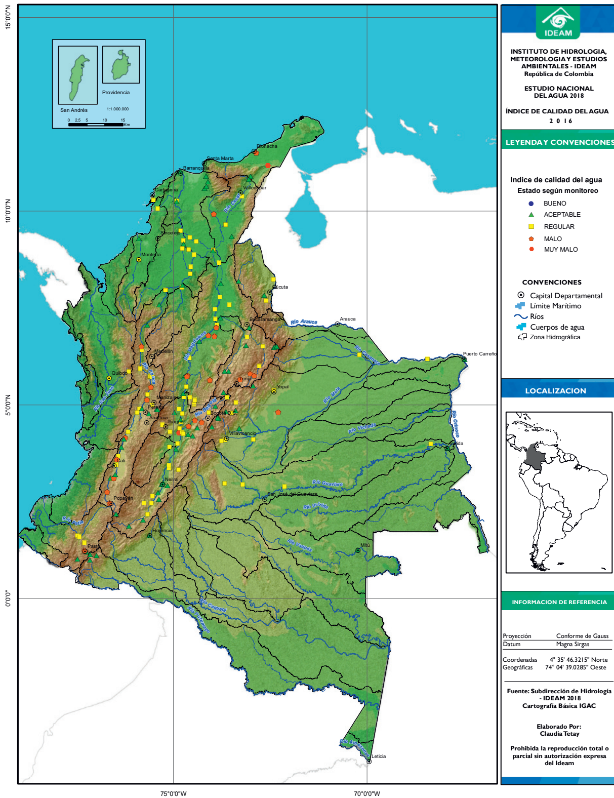
● Figura 123. Índice de calidad del agua 2016.
