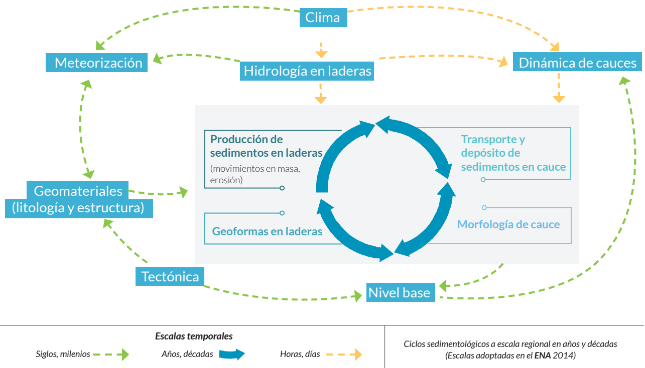
• Figura 49. Componentes del ciclo de sedimentos en diferentes escalas temporales y espaciales. Fuente: tomado del ENA 2014, modificado de (Preston & Schmidt, 2003).
