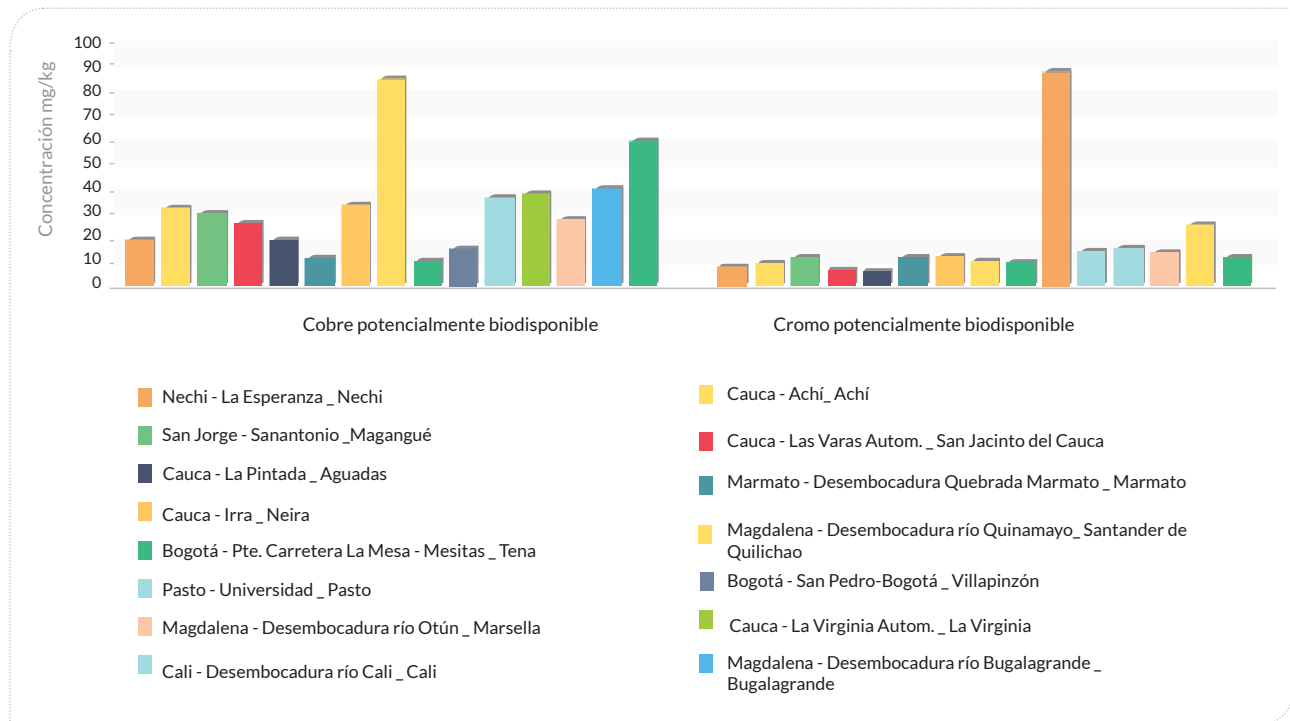
• Figura 114. Concentración de cobre (Cu) y cromo (Cr) potencialmente biodisponible.
