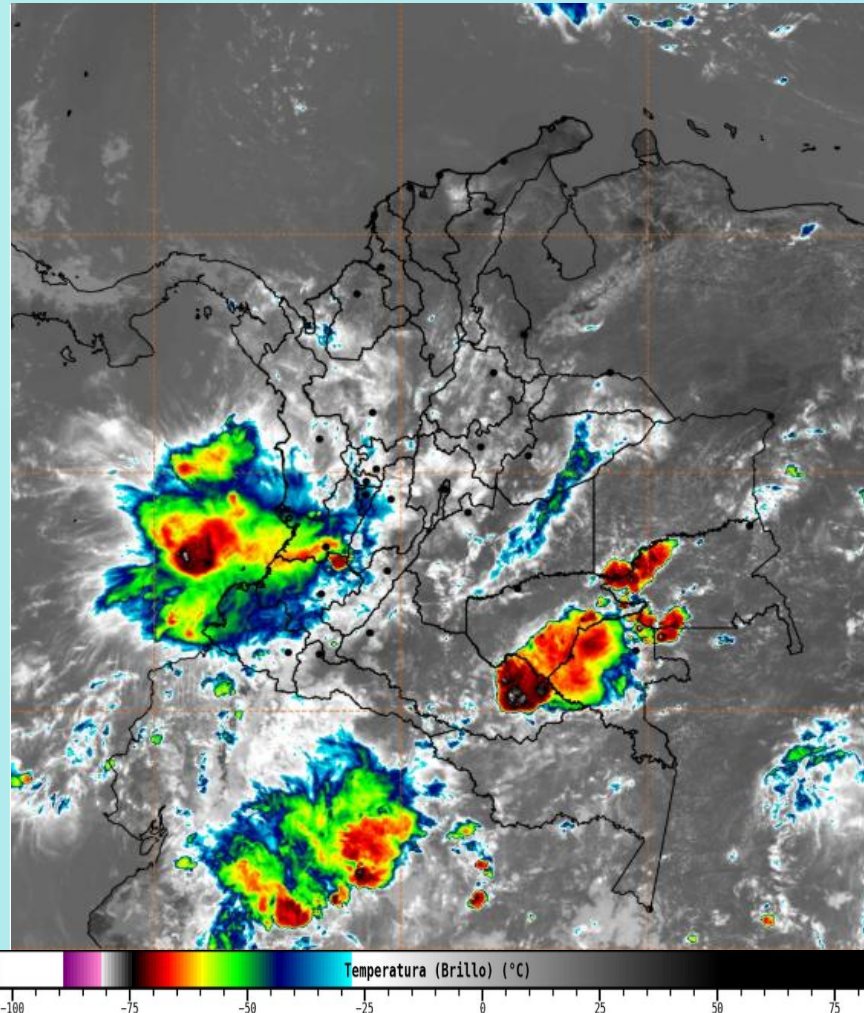
Imagen GOES 19 East Canal Infrarrojo, 29 de octubre de 2026 - Hora 12:00 HLC. Fuente: https://bart.ideam.gov.co GOES 19
