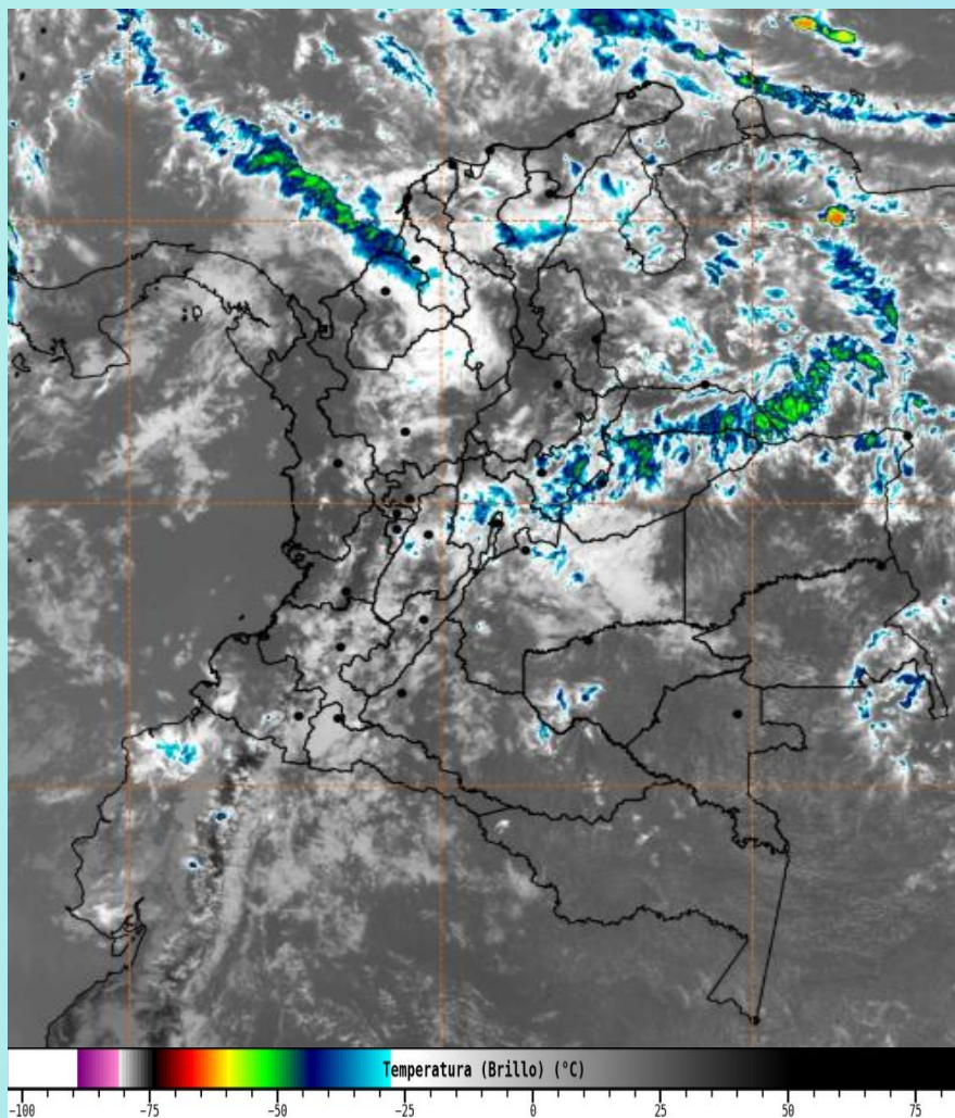
Imagen GOES 19 East Canal Infrarrojo, 04 de octubre de 2026 - Hora 11:50 HLC. Fuente: https://bart.ideam.gov.co GOES 19
