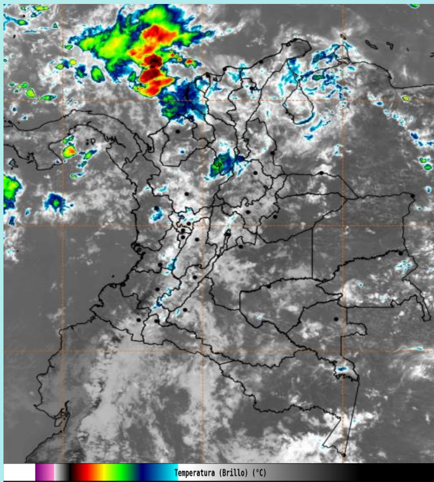
Imagen GOES 19 East Canal Infrarrojo, 28 de septiembre de 2026 - Hora 12:00 HLC. Fuente: https://bart.ideam.gov.co GOES 19
