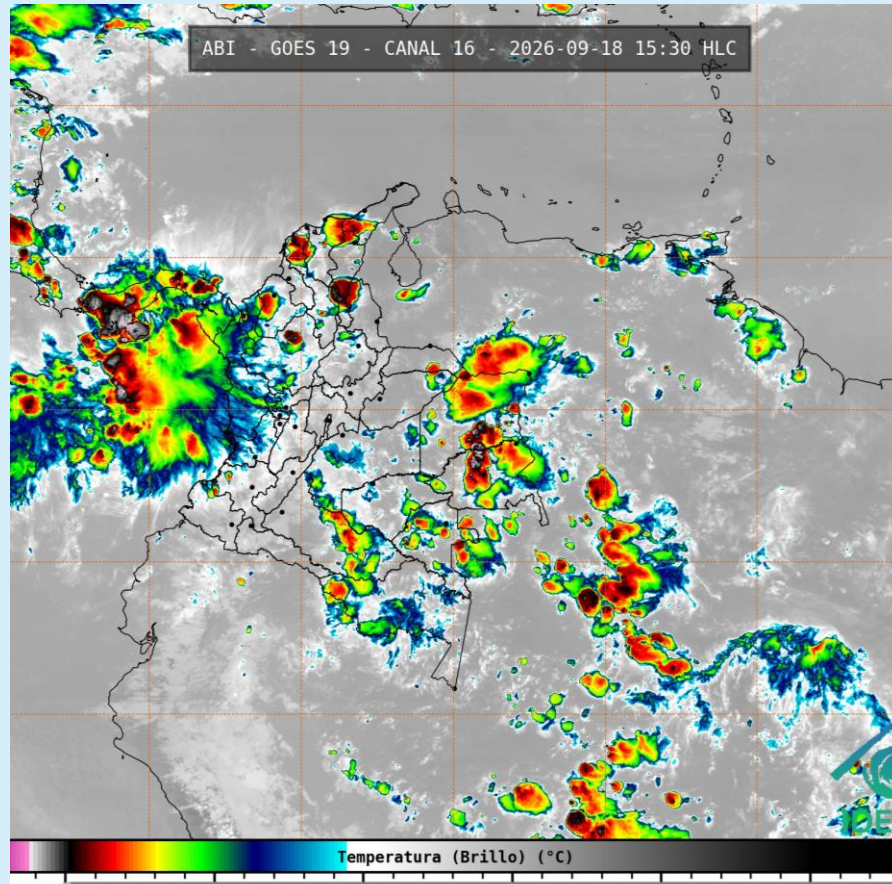
Canal Infrarrojo 18 de septiembre de 2026– Hora 15:30 HLC Fuente: GOES 19
