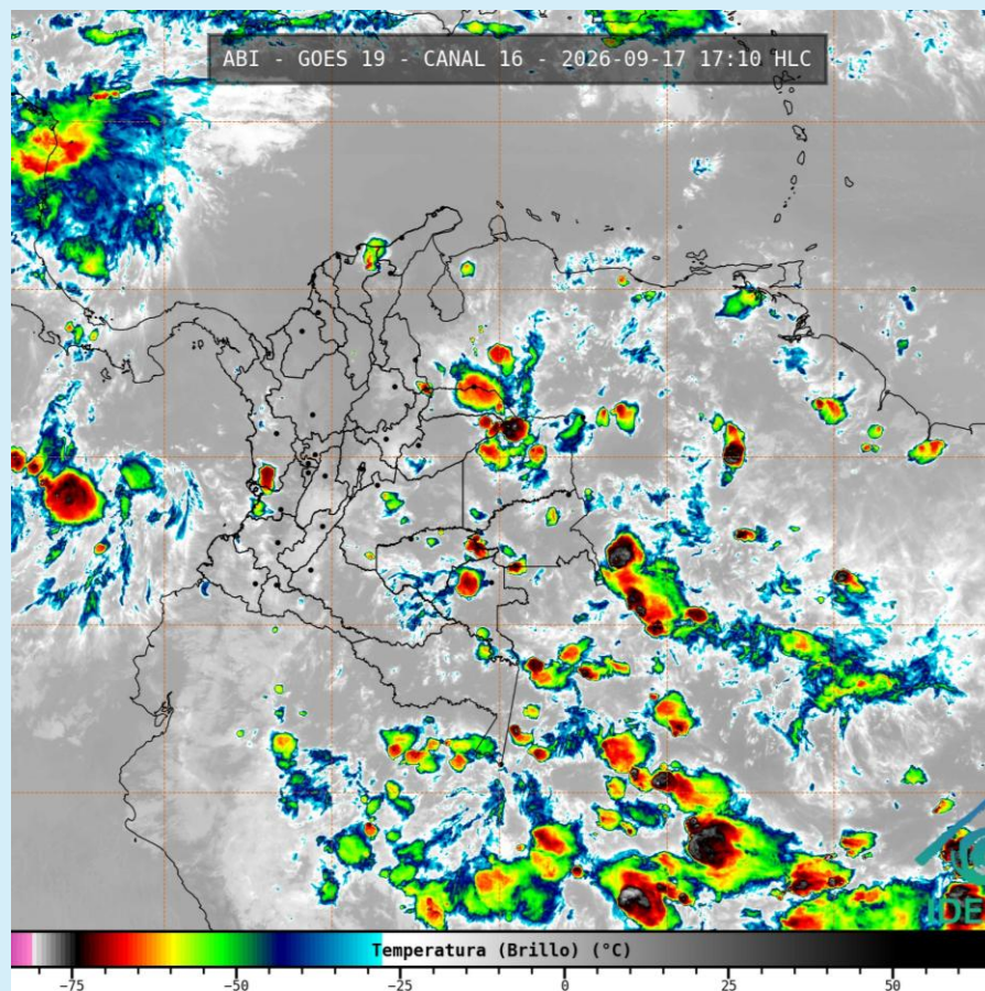
Canal Infrarrojo 17 de septiembre de 2026– Hora 17:10 HLC Fuente: GOES 19
